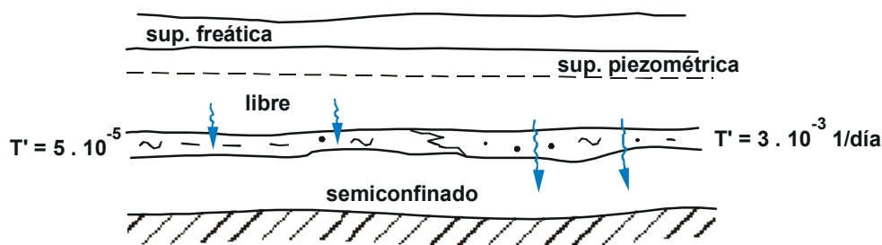
Flujo a través del acuitardo por variación de la transmisividad vertical
